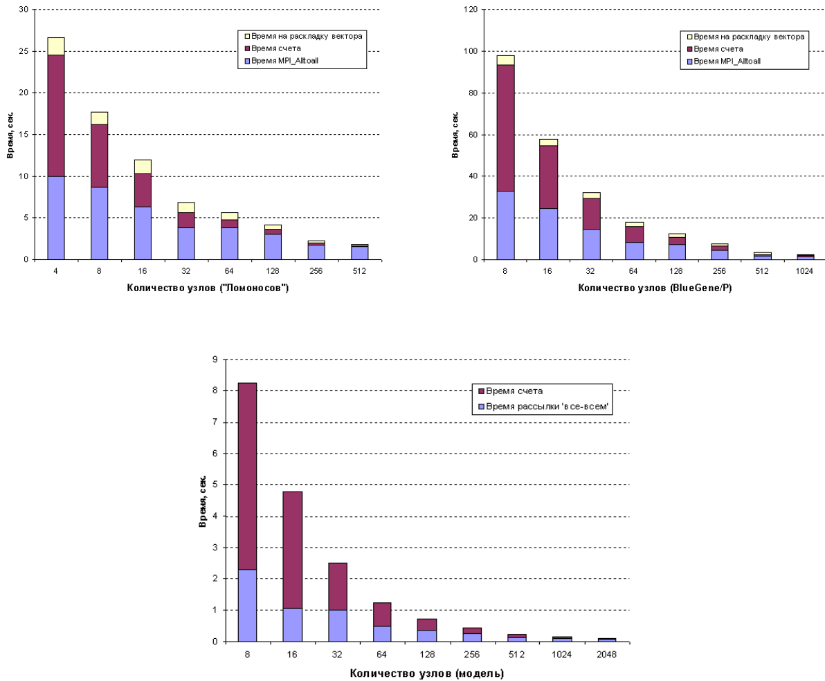
Рис. 2. Профиль выполнения 100 итераций третьего алгоритма «Alltoall» умножения разреженной матрицы на вектор ( n=10240000 , d=10 ) на суперкомпьютерах «Ломоносов», IBM BlueGene/P и на модели разрабатываемой коммуникационной сети.
